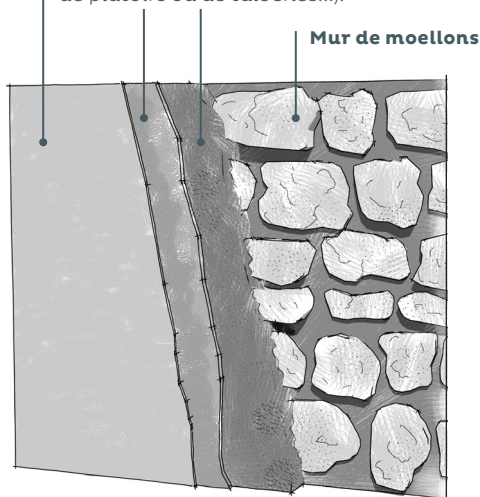
Les 3 couches d'un enduit à la chaux
